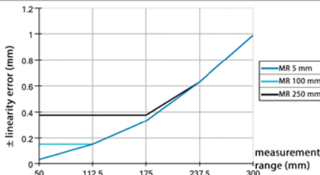
LAS-T-250, LAS-T5-250
