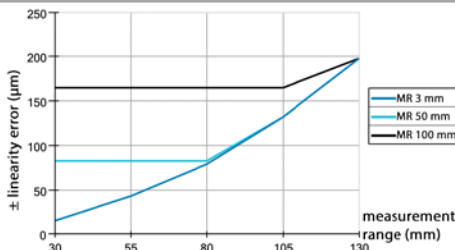
LAS-T-100, LAS-T5-100
