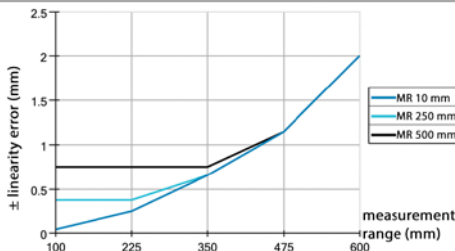
LAS-T-500, LAS-T5-500
